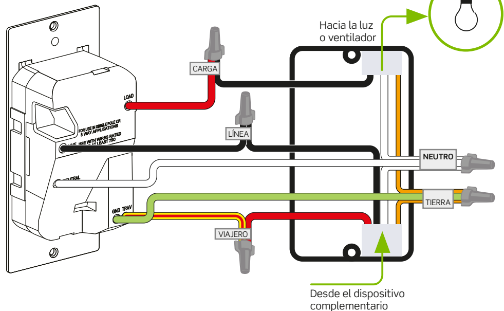
Atenuador complementario Cat. Núm. DD00R
