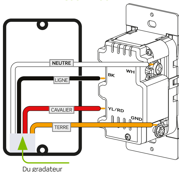
Gradateur complémentaire Cat. DD00R
