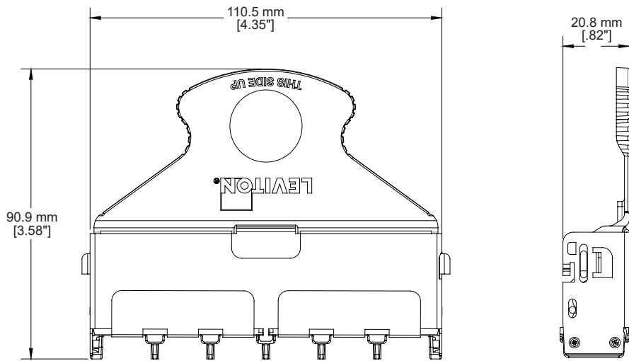
e2XHD Cassette
