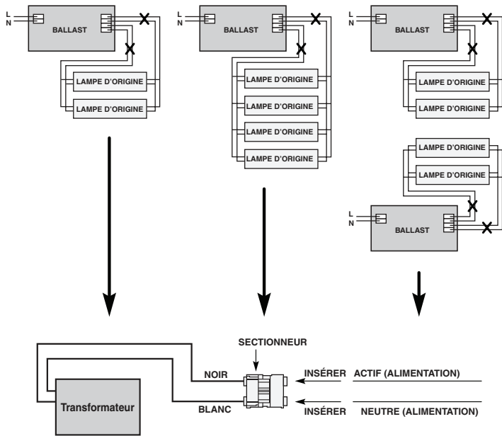
Diagramme simplifié d'un transformateur simple 60,96 cm x 60,96 cm (2' x 2') ou 60,96 cm x 1,22m (2' x 4')
