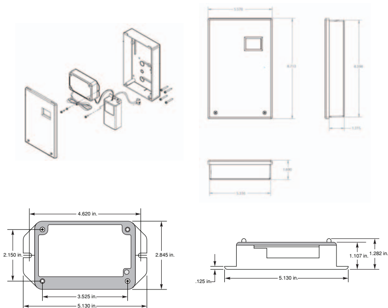
Figura 1 – Dimensiones del Medidor en Caja de Montaje en Superficie
