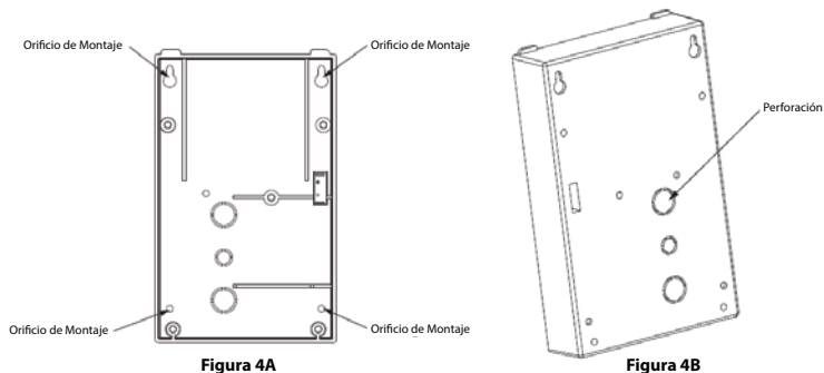
Figura 4A y 4B – Ubicaciones de los Orificios de Montaje
