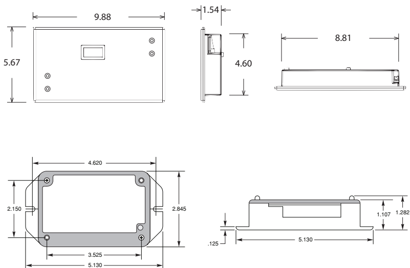
Figura 1 – Dimensiones de la Caja de Montaje Empotrado del Medidor Mini
