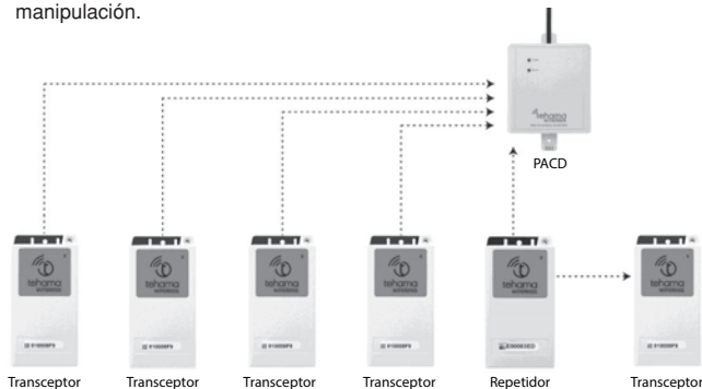
Figura 6 - Red Inalámbrica formada por TDMs, Repetidor, PACD
