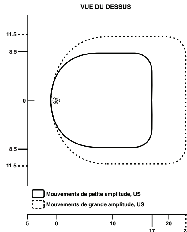
Figure 2 (N° de cat. OSC05) Champs de vision
