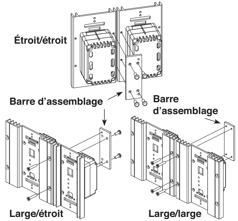
Figure 5 - Barre d'assemblage
