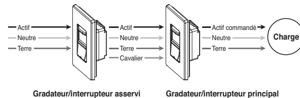
Schéma de câblage pour la commande à plusieurs voies
