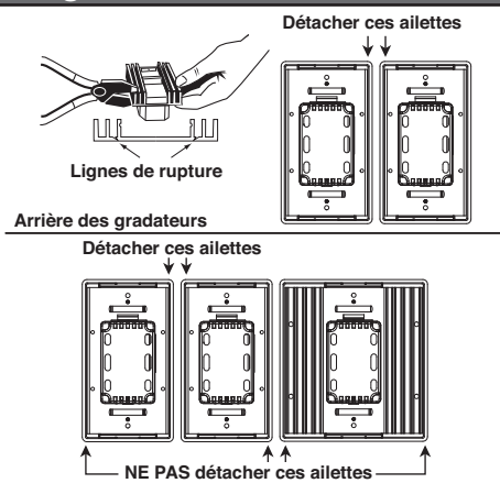
Figure 4 - Retrait des ailettes
