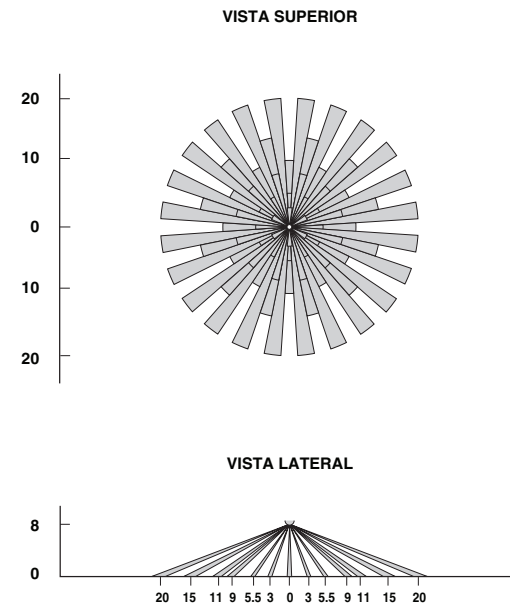
Figura 6 - (No. de Cat. O4C15) - Rangos Campo de visión Lente de largo alcance (marco negro), altura de montaje (8-12 pies)
