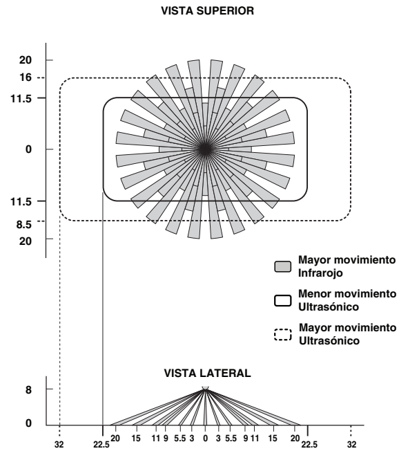
Figura 5 (No. de Cat. O4C20) Rangos Campo de Visión
