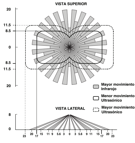
Figura 4 (No. de Cat. O4C10) Rangos Campo de Visión
