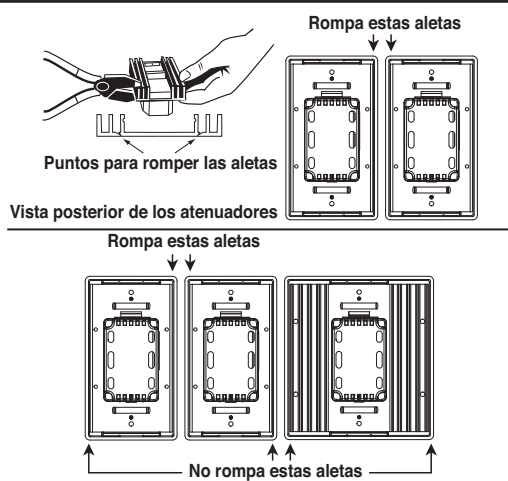
Figura 4 - Aleta Rota
