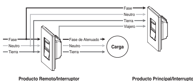
Carga entre el Producto Remoto/Interruptor y Producto Principal/Interruptor
