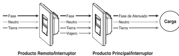
Carga después del Producto Remoto/Interruptor y Producto Principal/Interruptor
