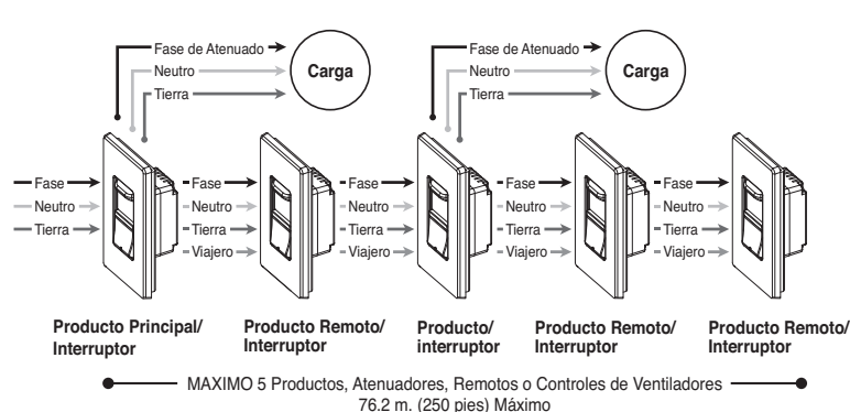
Productos Múltiples/Interruptor y Producto Principal/Interruptor Remoto
