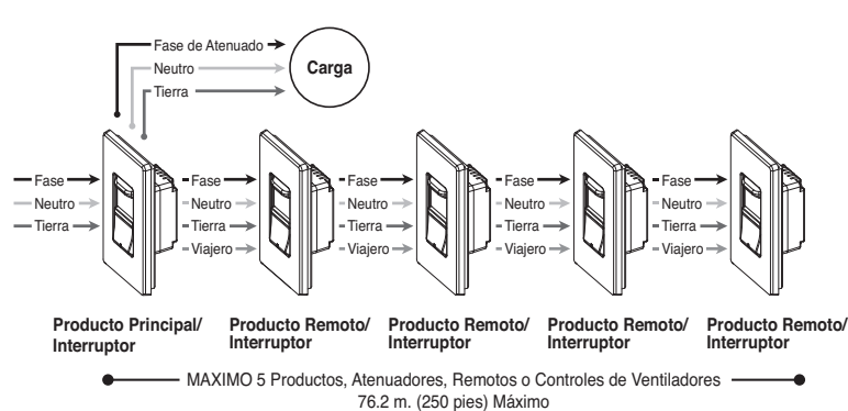
Producto Remoto/Interruptores Múltiples
