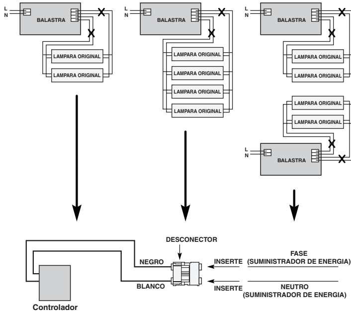
Esquema Simple del Control 60 cm x 60cm y 60 x 1.20m (2' x 2' y 2' x 4')
