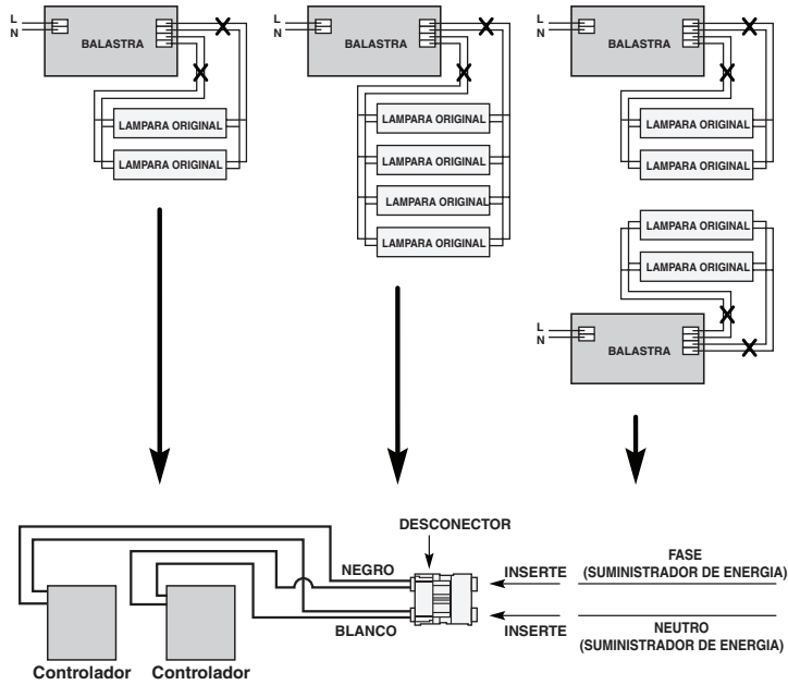
Esquema Doble del Control 60 cm x 60cm y 60 x 1.20m (2' x 4')
