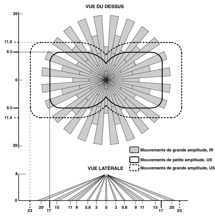
Figure 3 (N° de cat. OSC10) Champs de vision
