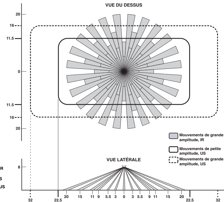
Figure 4 (N° de cat. OSC20) Champs de vision
