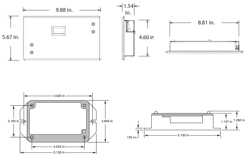
Figure 1 — Dimensions d'un compteur en boîtier affleurant
