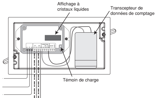
Figure 2 — Connexions et affichage des compteurs
