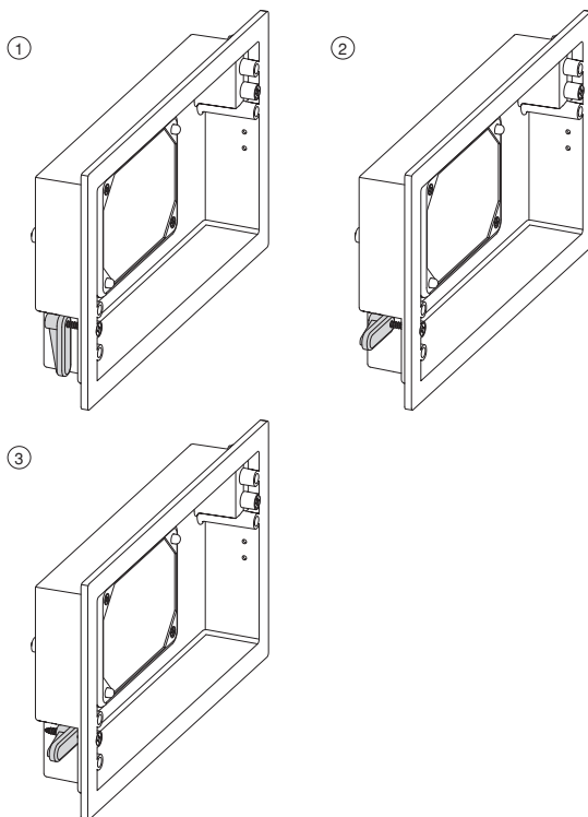
Figure 4 — Installation du boîtier affleurant
