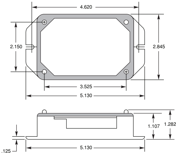
Figure 1 – Dimensions d'un minicompteur, en pouces
