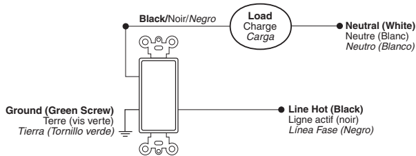
Wiring Diagram/Schéma de câblage/Diagrama de Cableado
